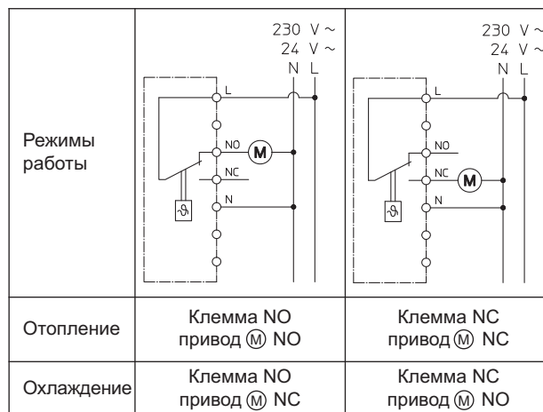
Схема подключения
